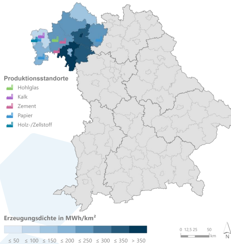
Stromerzeugung für PV und Wind in Unterfranken 2019
