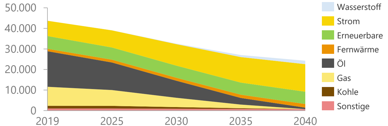
Entwicklung des Endenergieverbrauchs inkl. stofflicher Nutzung in GWh | Unterfranken | Szenario E.Plan
